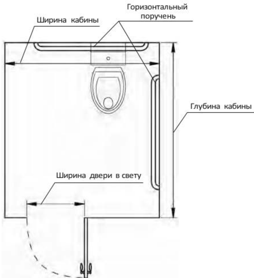
Рис. 5. Санитарно-гигиеническое помещение
